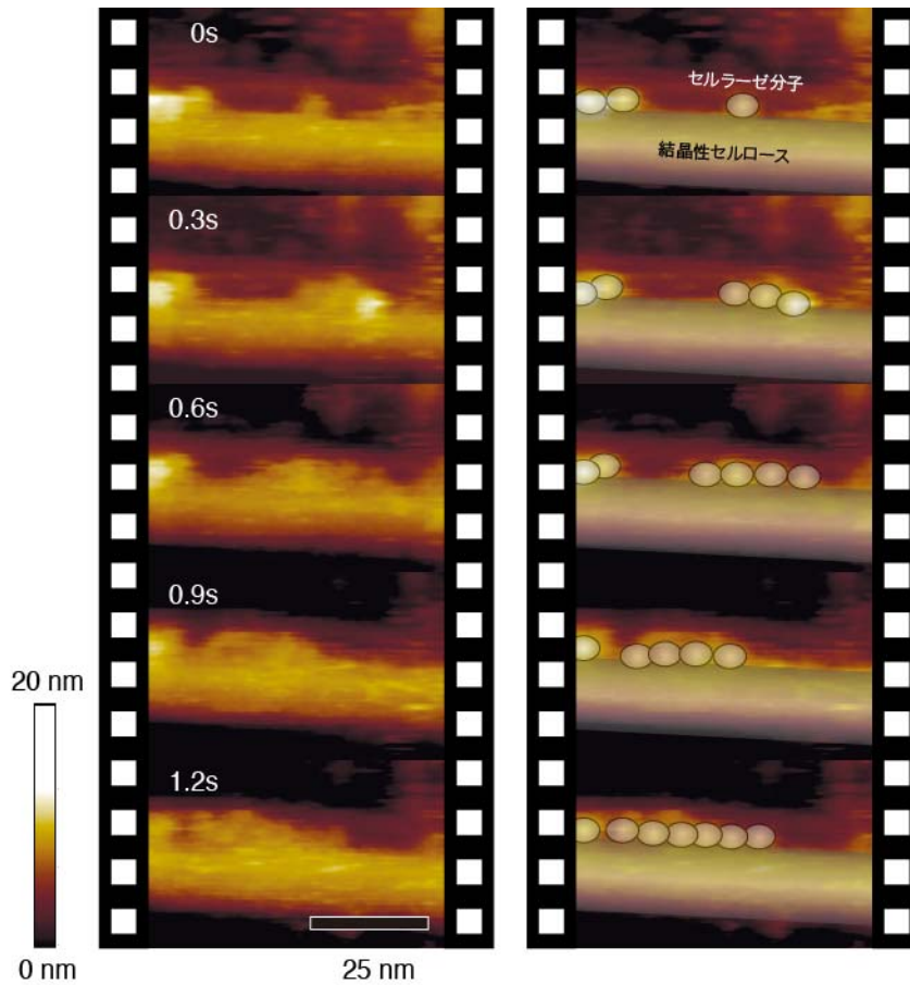
(図1) セルラーゼがセルロース結晶表面を一方向に進みながら分解していく様子。
