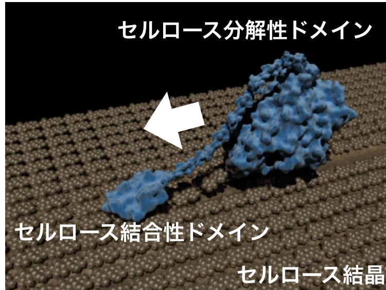
(図1) セルラーゼがセルロース結晶表面を一方向に進みながら分解していく様子。
