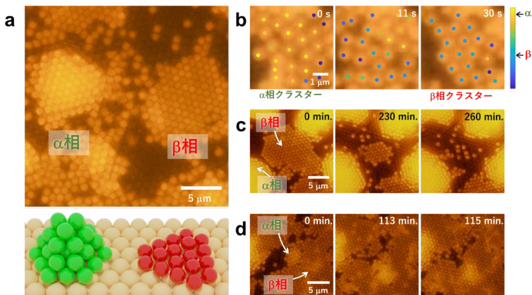
図 1. (a) ヘテロエピタキシャル成長により得られた結晶多形の顕微鏡像および模式図（α相：緑色，β相：赤色）。粒径 860 nm のポリスチレン粒子をエピタキシャル相、1300 nm を基板結晶に使用。(b) 核形成における多形転移のスナップショット。(c) 結晶成長中に起きる溶液を媒介して発生するβ相からα相への多形転移のスナップショット。(d) 結晶成長中に起きる固体のα相から固体のβ相への多形転移のスナップショット。
