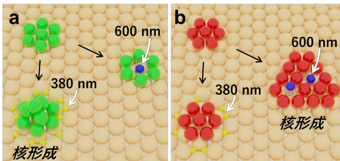
図 2. 異なる粒径の粒子添加 (380 nm と 600 nm) による多形制御の模式図。各多形の形状の違いにより、クラスターの核形成が阻害される添加粒子の粒径が異なる。(a) α相は置換型の添加粒子 (600 nm) によってクラスターの核形成が阻害される。(b) β相は基板と結晶の間に入ってくる添加粒子 (380 nm) によってクラスターの核形成が阻害される。
